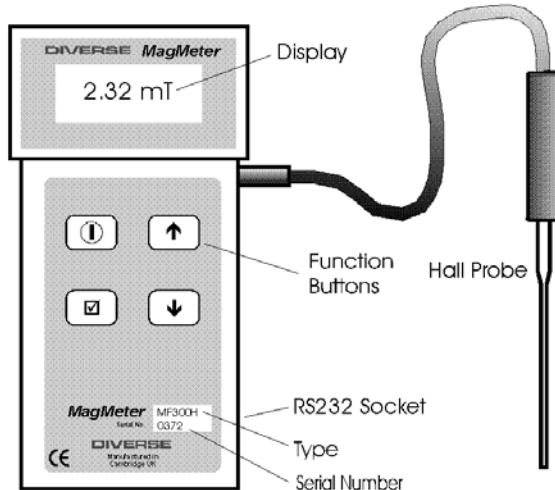
Fig. 2 MF300H MagMeter
