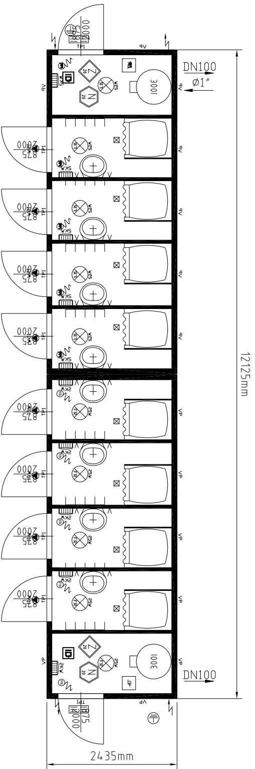
601858.dwg
